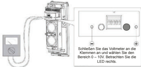
Abb. 6 Einstellung mit Voltmeter
