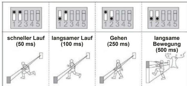
Abb. 7 Einstellung der Reaktionszeit
