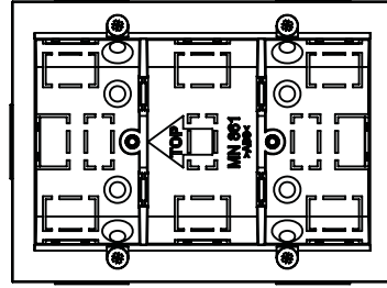
S Montážní otvor Mounting hole X=70/Y=96
