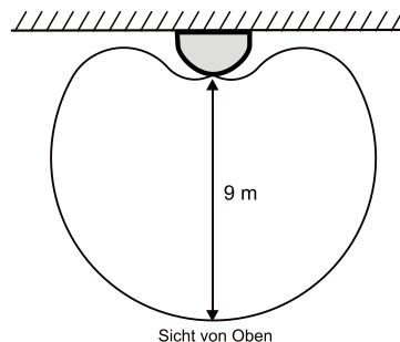
Erfassungsbereich des Glasbruchsensors
