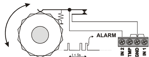
Beispiel des Anschließens des Eintrittes IN2
