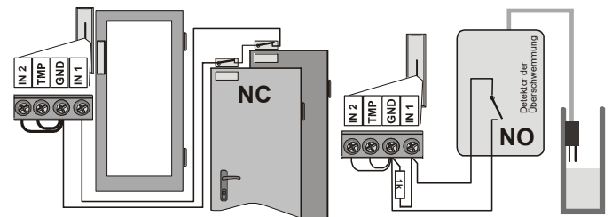
Beispiel des Anschließens der externen Sensoren mit dem Trenn- und Schaltkontakt
