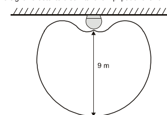
Záběrová charakteristika detektoru rozbití skla
