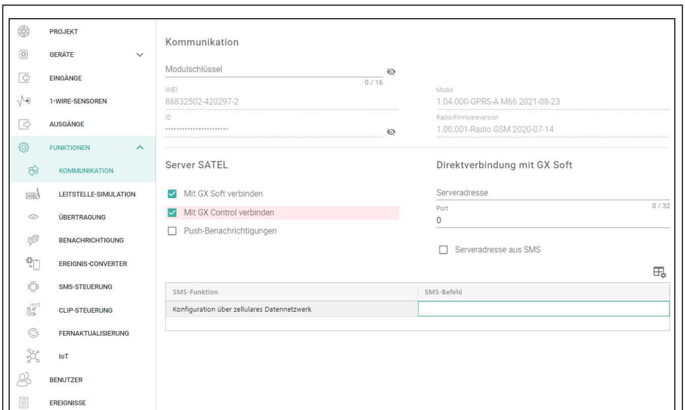
Abb. 24. Registerkarte „Kommunikation“.
