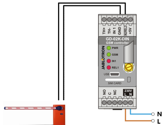
Abbildung 2: Tor-Controller GD-02K-DIN.
