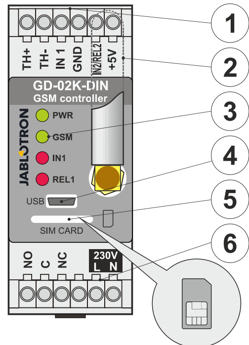
Abbildung 1: 1 – Niederspannungsklemmen; 2 – GSM-Antenne; 3 – LED-Anzeigen; 4 – MicroUSB-Anschluss zur Verbindung mit einem PC; 5 – SIM-Karteneinsatz; 6 – Stromausgangsrelaisklemmen und 230 V Stromklemmen.
