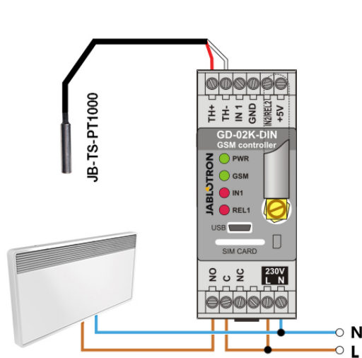
Abbildung 5: Temperaturüberwachung und Heizsteuerung. R – rotes Kabel; W – weißes Kabel
